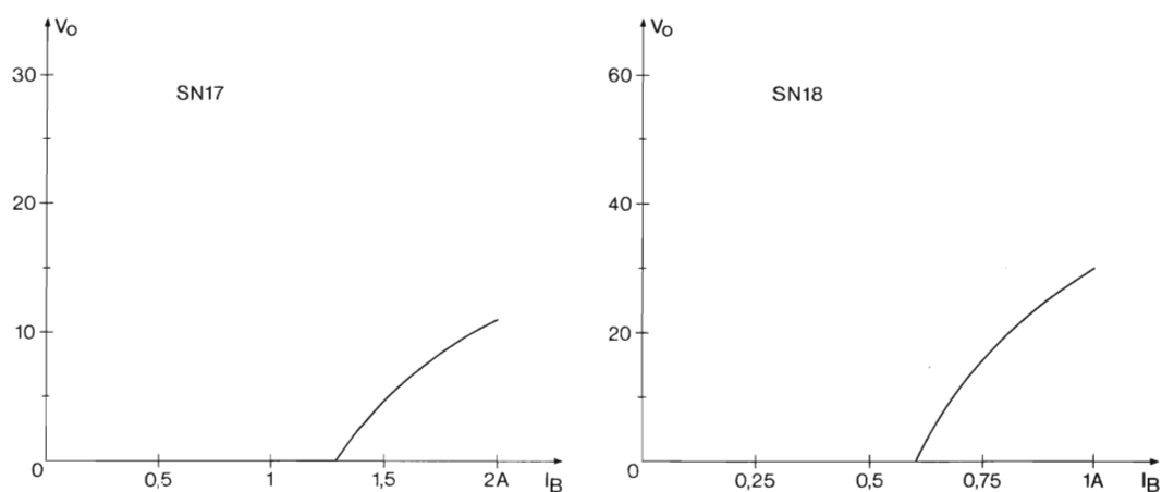
Fig. 12. Belastningskarakteristik for SN17/18
