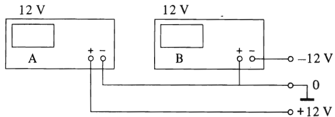
Fig. 10. Bipolar spændingsforsyning.
