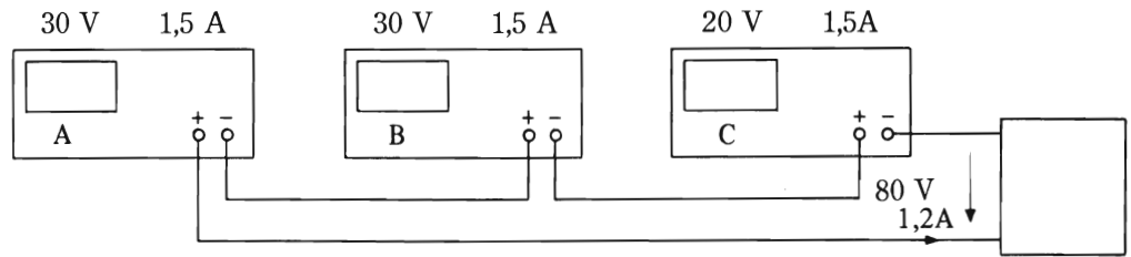
Fig. 9. Serieforbindelse af tre SN17-enheder
