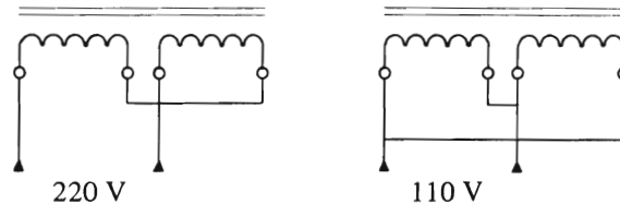
Fig. 1. Ændring til 110 V netspænding.
